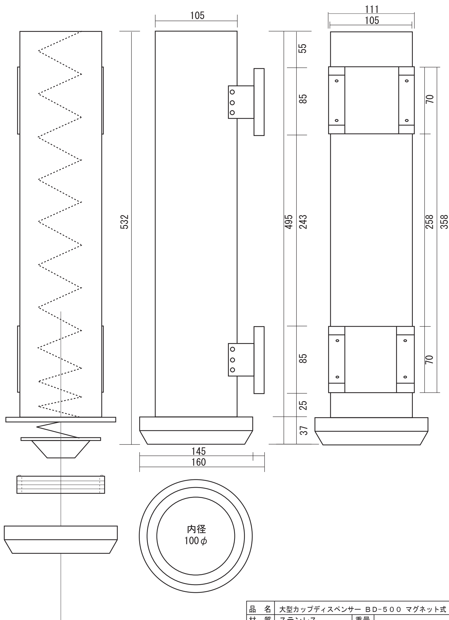
大型カップディスペンサー BD-500 寸法図
