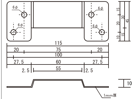
上部引掛けフック
