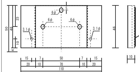
下部固定フック
